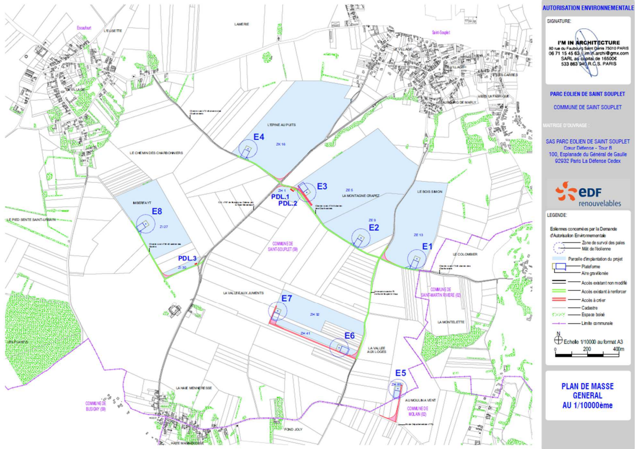
Carte 2 Plan en phase exploitation du parc éolien de Saint-Souplet (I'm In Architecture)
